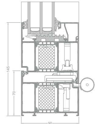
řez dveřmi STAR
