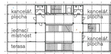
Půdorys 3. NP
