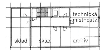
Půdorys 1. PP
