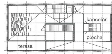
Půdorys 4. NP
