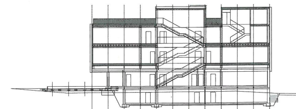
Řez podélný
